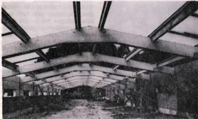
Perutninarska farma Hajnsko — prvi tak objekt po montažnem sistemu Ingrad
