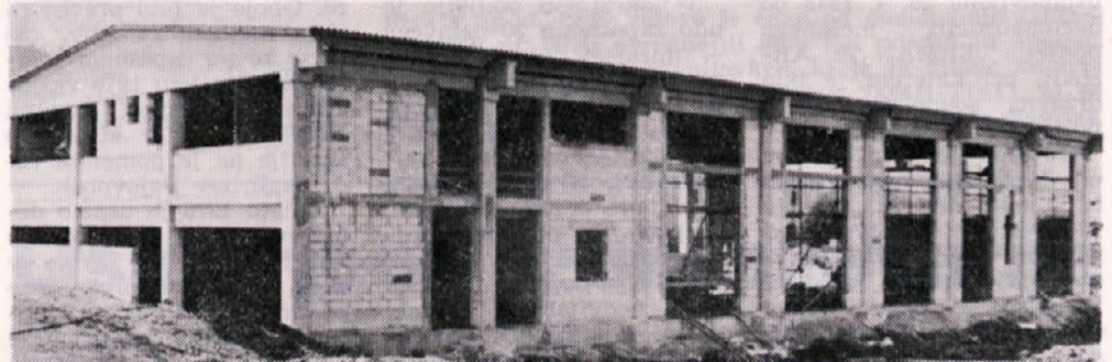
Avtomehanično delavnico za celjsko Cinkarno gradimo po montažnem sistemu Ingrad
