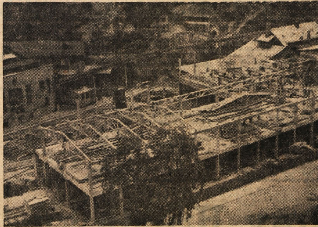
DEL KONSTRUKCIJE PRI REKONSTRUKCIJI HRASTNIŠKE STEKLARNE. DELO NAGLO NAPREDUJE IN VIDITI JE, DA BO PRVA ETAPA KONČANA V PREDVIDENEM ROKU
