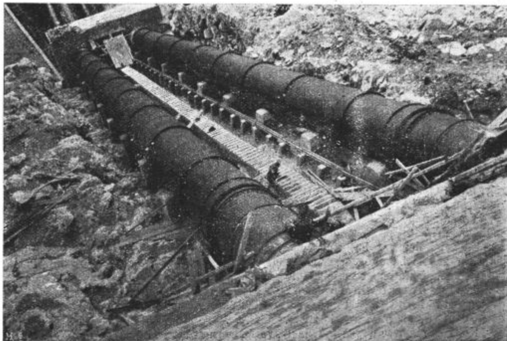
Podoba 76. Omiške tvornice: Cevasti vodovodi pri centrali sil v Kraljevaču.
