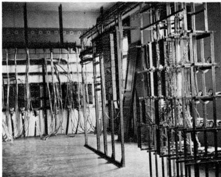
Dvorana kablov: Preiskovalna dvorana za medkrajevne in lokalne telefonske proge.
