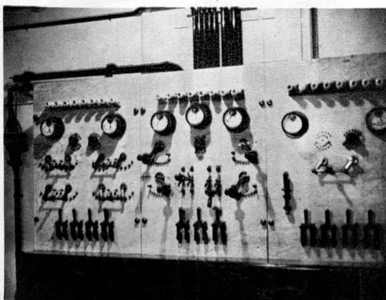
Stikalna plošča za polnjenje brzojavnih akumulatorjev.
