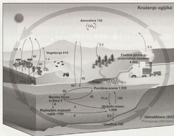
Kroženje ogljika
