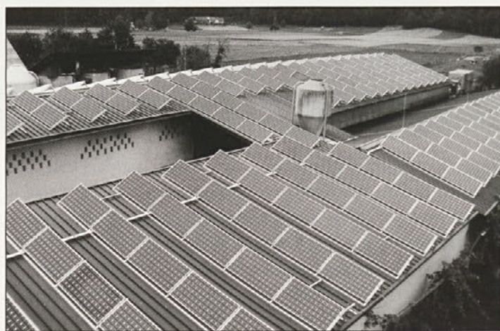
Sončna elektrarna na kmetiji Muzek v Zg. Pristavi zavzema 276 monokristalnih panelov, skupne moči 49,68 kW.
