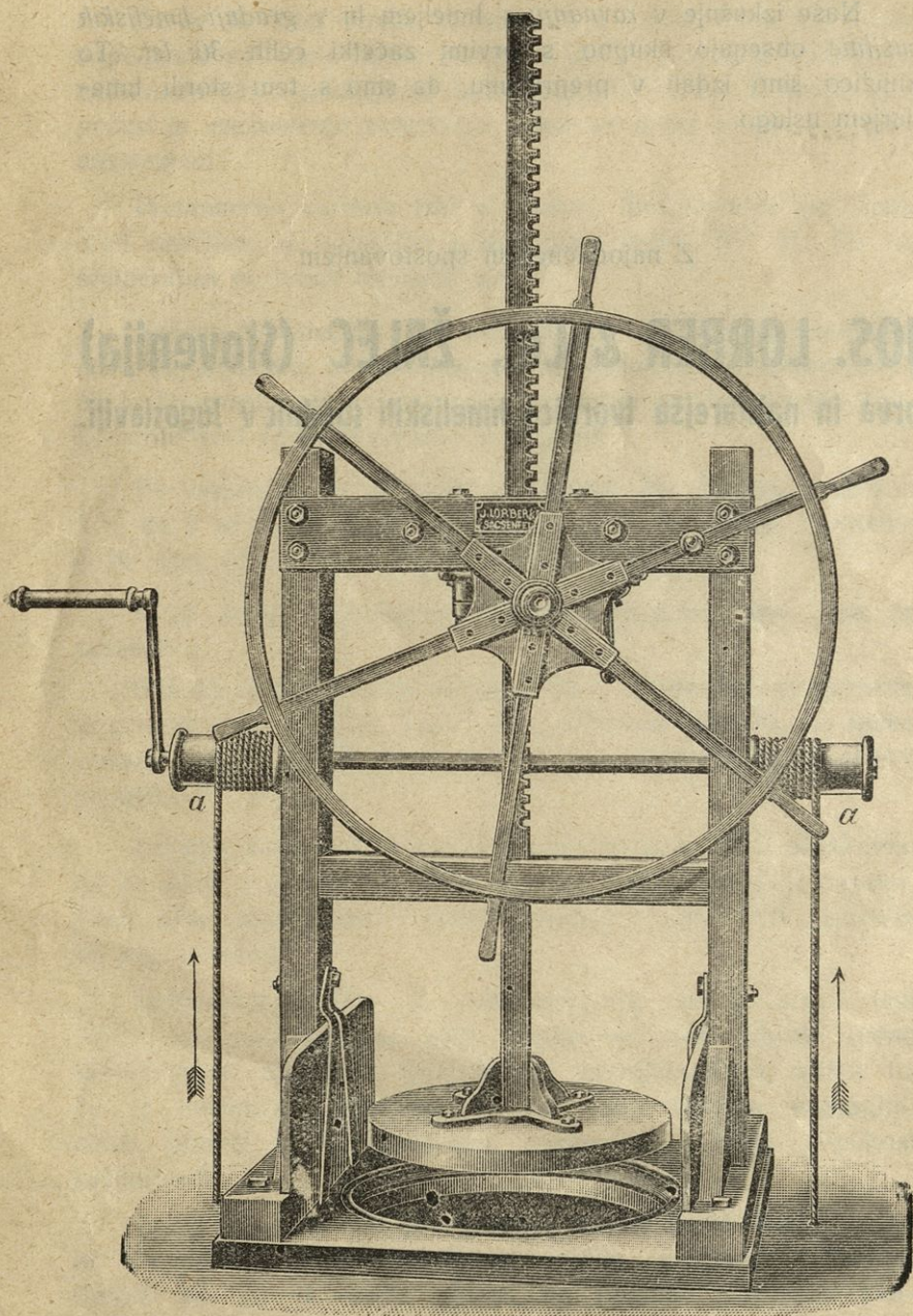
Hmeljska stiskalnica sistema »Lorber«.
