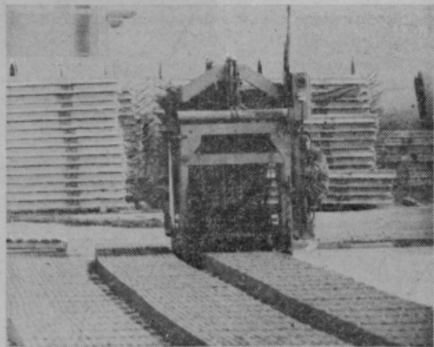
Proizvodnja opažnih votlakov
