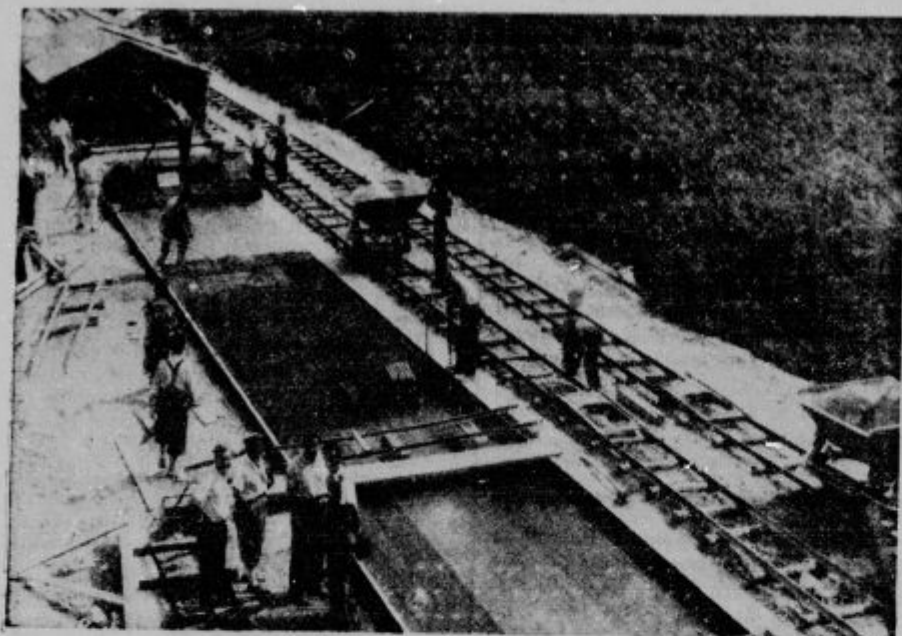
Pogled na celotni postopek betoniranja betonske ceste. Spodaj je s papirjem pokrito cestišče.
