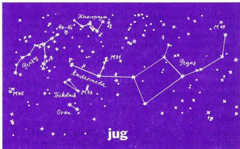
Slika 1. Ozvezdje Pegaz, v njem zvezda Nos in kroglasta kopica M 15. Fizikalne karakteristike zvezde in kopice poiščite v kakem zanesljivem priročniku, na primer v Karti severnega in južnega neba , ki je izšla pri DMFA Slovenije, ali v kakšnem računalniškem programu.
