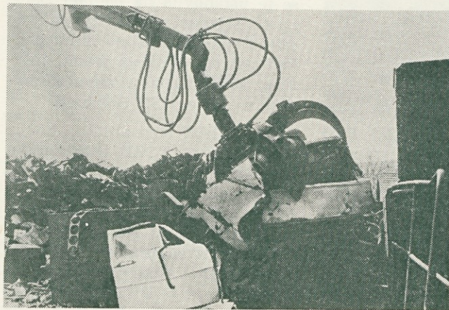
Grabilec dvigala LIV je še zadnjič potisnil karoserijo Škode nad odprtino za stiskanje
