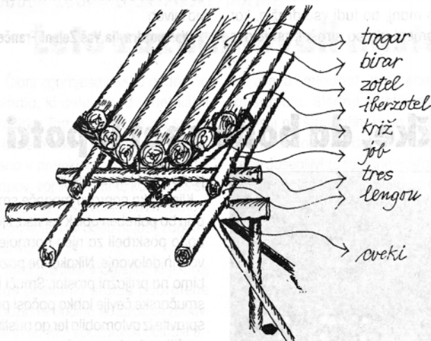
Med številnimi cveki je bil "tumpel" vezni člen med trami v riži, če je ta peljala v zavoju. Tam je bila največja nevarnost, da les raztrga rižo.
