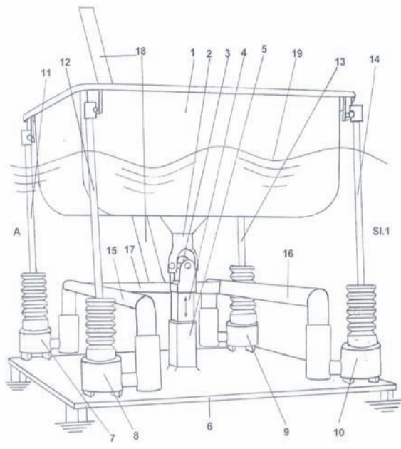
Skica in prototip naprave za izrabo energije morskega valovanja. Celotna naprava naj bi stala v vodi, razen dveh tretjin plavajoče ponve. Ta se giblje v vse štiri smeri in tudi vertikalno, s čimer se prilagaja plimi in oseki. Ponev služi za poganjanje tlačilk, ki vodo po cevovodu potiskajo v akumulacijski bazen na obali. Ko se voda vrača v morje in pri tem teče skozi turbinski sistem, se ustvarja električna energija.
