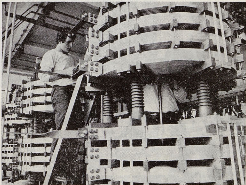
Revizija naprave za kompenzacijo jalove električne energije
