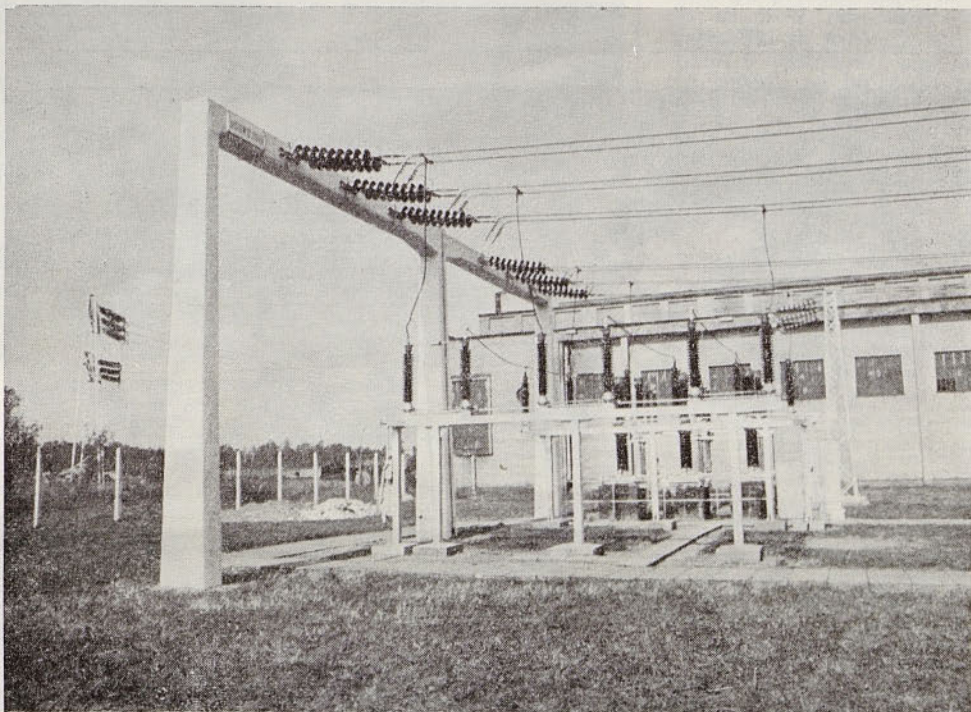
RTP Kidričevo po rekonstrukciji
