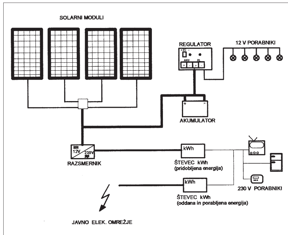
Slika št. 4: Shema sistema povezanega z javnim električnim omrežjem
