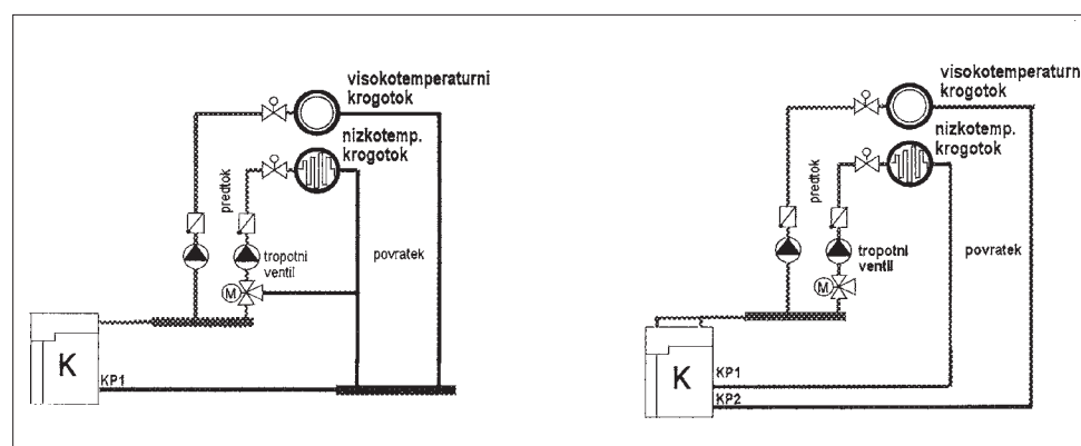
Slika 9: Vgradnja kondenzacijskega kotla za visokotemperaturne in nizkotemperaturne krogotoke
