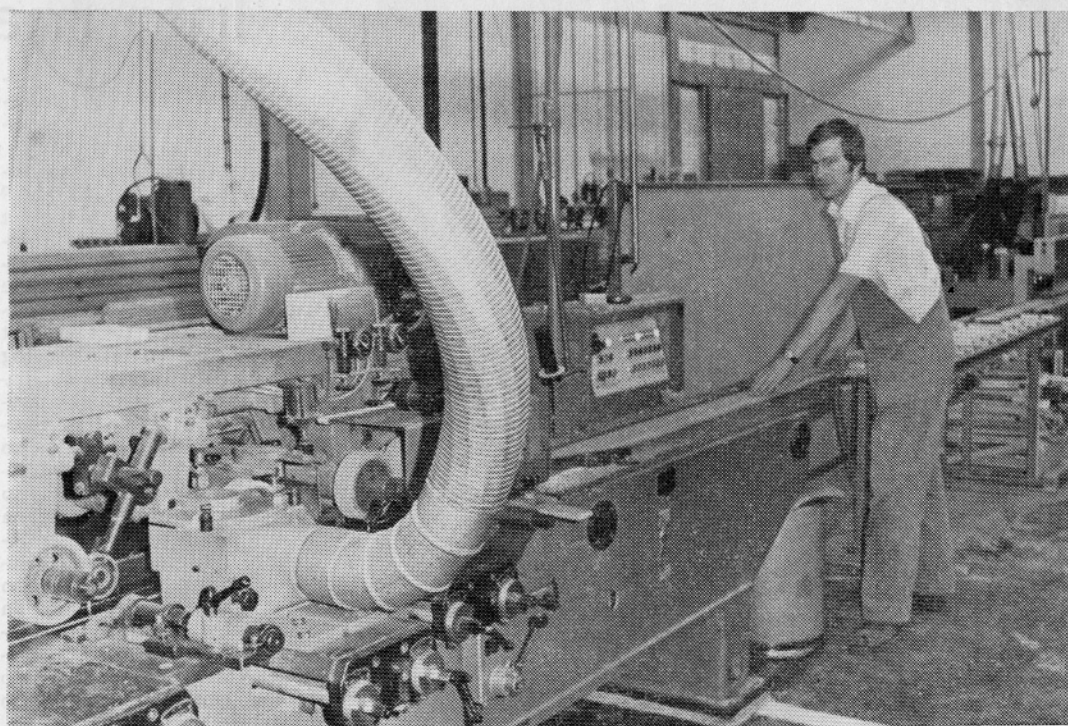
Profiliranje elementov za suhomontažni podboj TO Rečica (foto Ažman)
