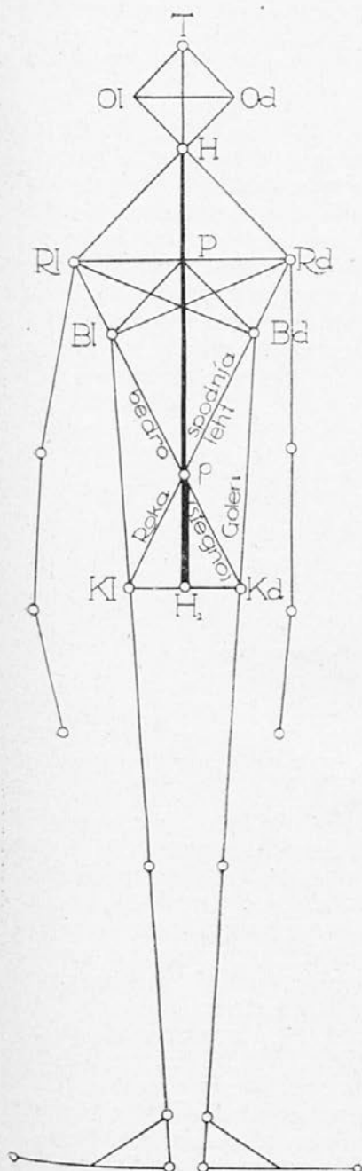
Obr. 1. Schmidt-Fritschev ključ.
