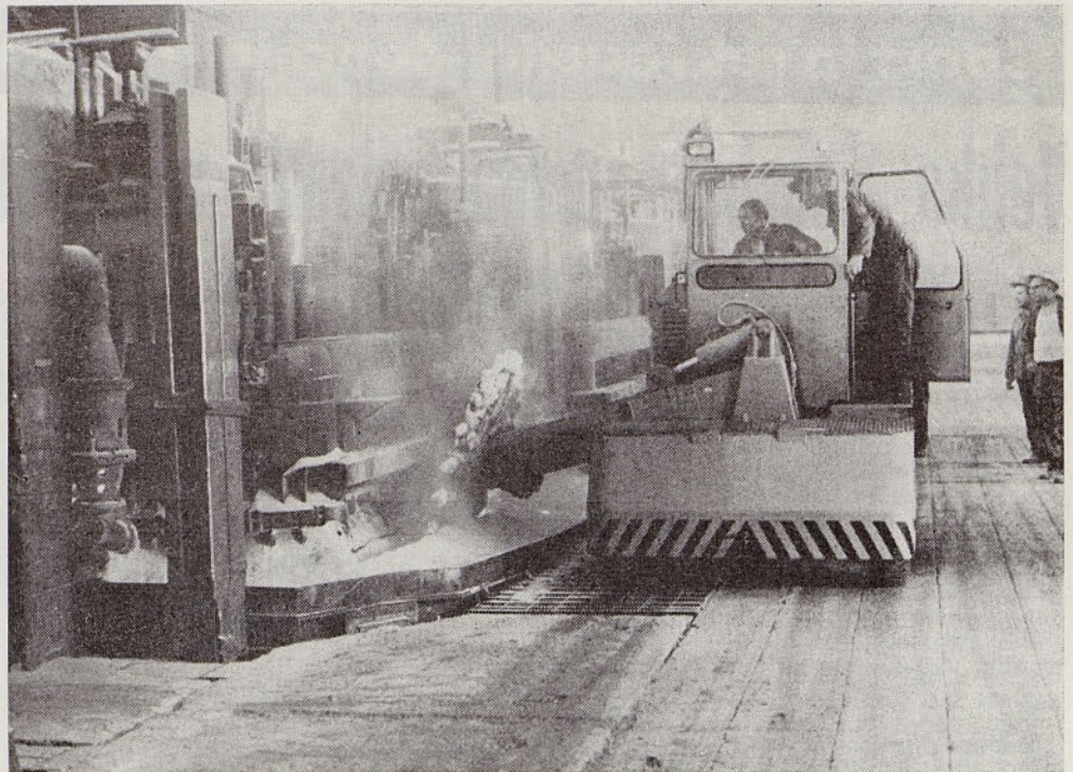
Pribjalni stroj s kolesom
