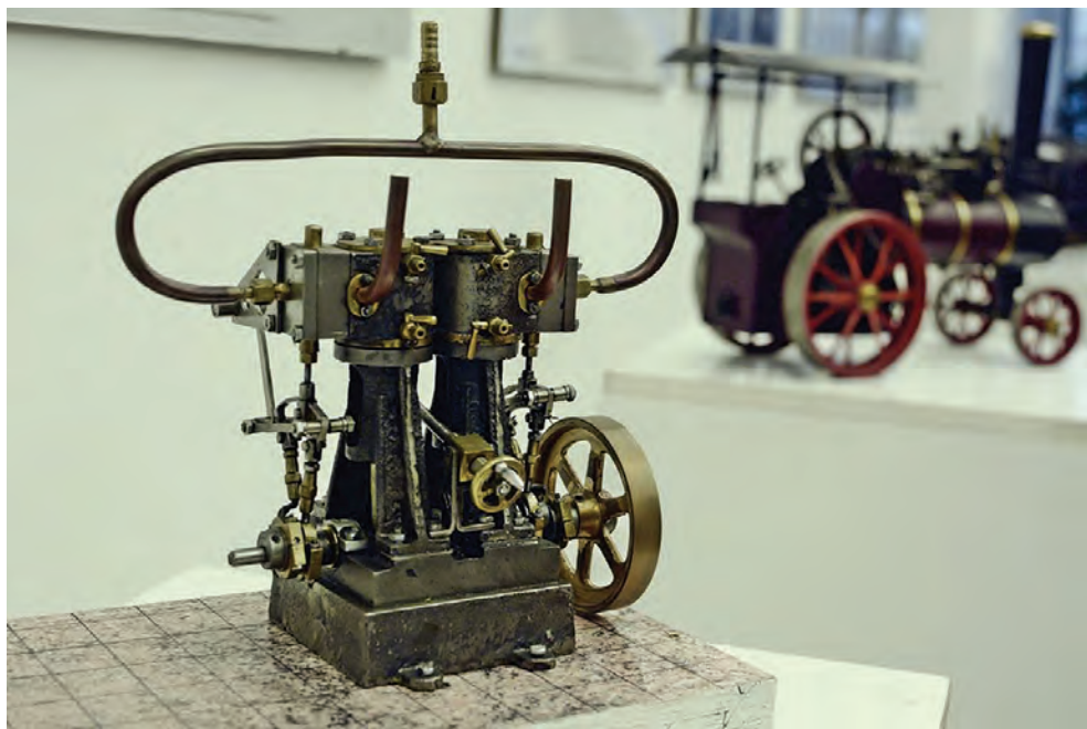
Ladijski parni stroj kot razstavni eksponat na razstavi v Avli Cankarjevega doma na Vrhniki. Merilo 1 : 10, 2014. Foto: Gašper Tominc.
