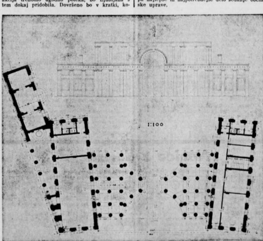
Veličastno pročelje »Vrta vseh svetnikov« po osnutkih prof. Plečnika, ki ga bo krasilo bogato stebrovje (po številu 104). Spodaj tloris pročelja in prostor ob vhodu. Desno od vhoda bodo poslovni prostori in prostori za duhovščino, na levi pa prostor za svetilce in polaganje mrtličev. — (Kapelice pa bodo razvrščene dalje po parku. Ograja okrog parka bo le deloma zidana, v glavnem pa jo bo tvorila dvojna živa meja.)
