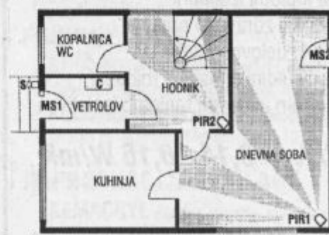
S - sirena C - centrala MS - magnetno stikalo PIR - infrardeči senzor
