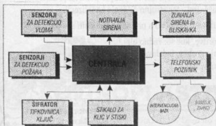
shema alarmnega sistema
