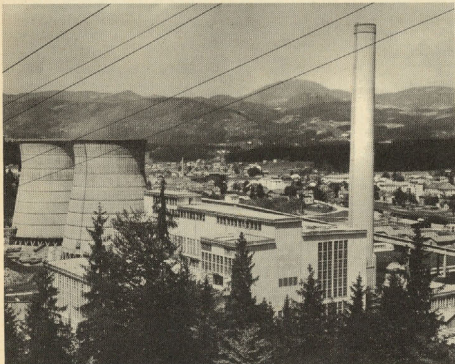
Pogled na TE Šoštanj leta 1960, ko je bila dokončana II. faza njene izgradnje.
