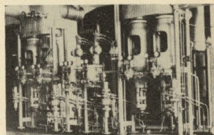
Posnetek iz leta 1955: Pomemben del sistema kotlovskih naprav v TE Šoštanj - oljna regulacijska črpalka!
