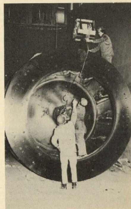
Pripravljen rotor enega od mlinov za premog v TE Šoštanj za transport v delavnico na popravilo
