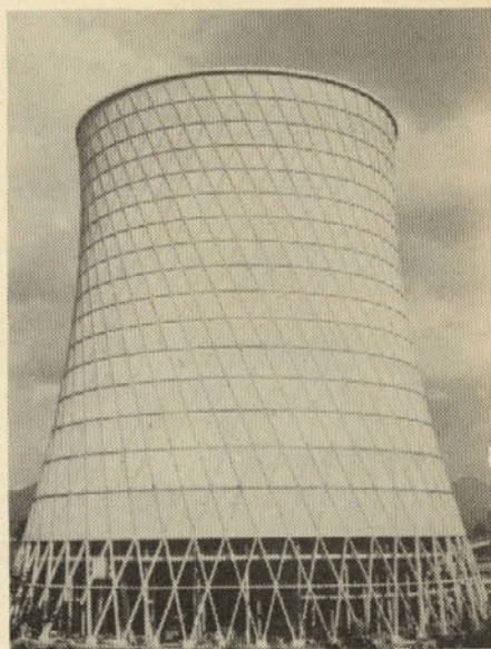
Posnetek iz leta 1976: Hladilni stolp v TE Šoštanj - sestavljen iz "nešteti" trikotnih betonskih elementov, visok 94 metrov in z zmogljivostjo ohlajanja 20 000 kubičnih metrov vode na uro - je dokončan!
