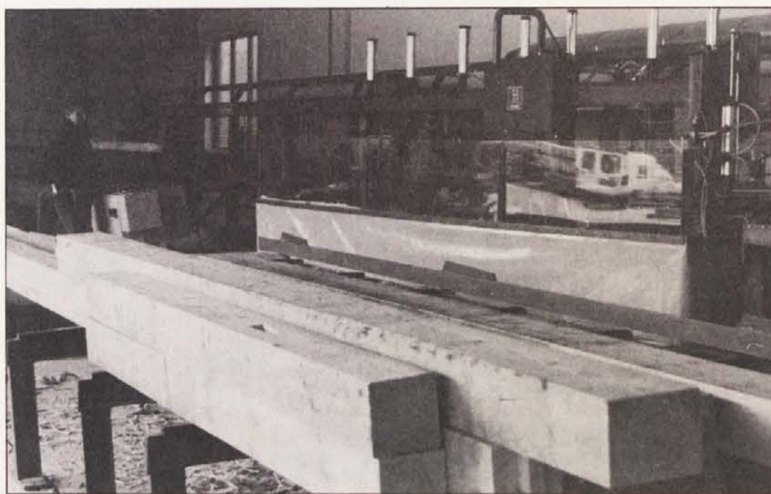
Podjetje Gasser s to napravo kompjutersko pripravi tramove za vezavo ostrešij.
