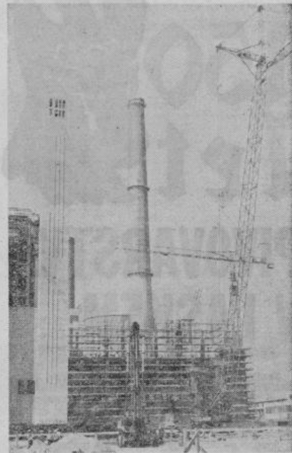
Soštanj. Graditev četrte faze termoelektrarne. Največje gradbišče, kjer sodeluje in dela izvaja kolektiv celjske enote Gradisa. Sicer pa, Gradis je tu že kar doma. Z gradbenimi deli je sodeloval pri postavitvi vseh dosedanjih faz elektroenergetskega giganta v Saleški dolini. In ne samo to — vsa dela je izvršil v dogovorjenih rokih. Na posnetku: bunkerski del in začetek del pri pilotiranju hladilnega stolpa. Ob kotlarni je zgrajeno tudi stopnišče.
