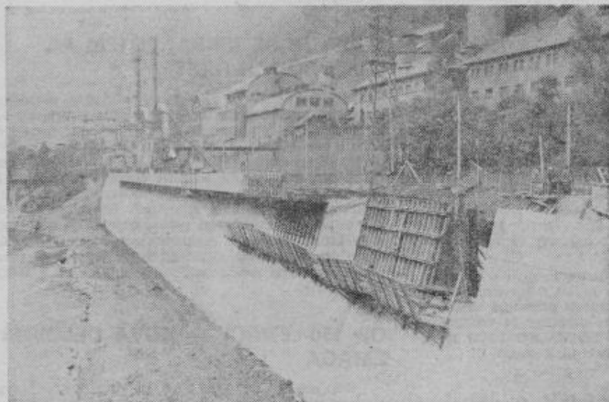
Oporni zid na bregu Save v Trbovljah. Izredno zahteven objekt. Tudi zaradi gradnje, zaradi nihanja vodne gladine, zaradi delovnih pogojev. V njem je 6.000 kubičnih metrov betona.
