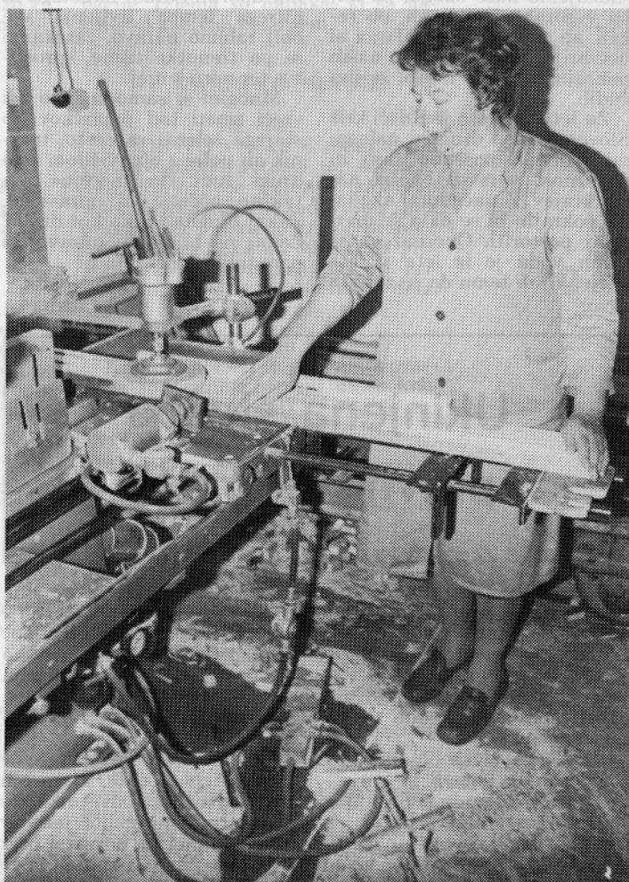
V TO Mojstrana - čepjenje in čeljenje elementov za skelete vhodnih in garažnih vrat
