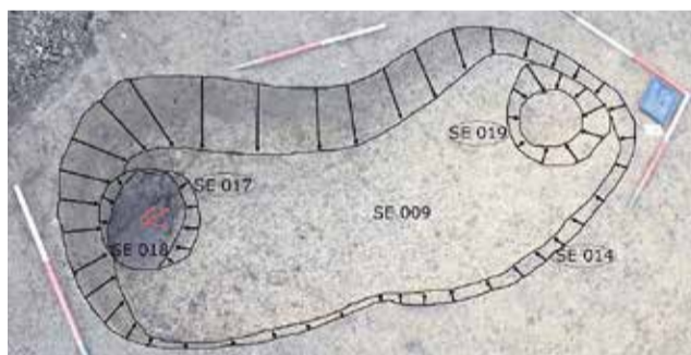
Tlorisni pogled na zemljanko z interpretiranimi plastmi po odstranitvi zasutja zemljanke; z oranžnimi puščicami je označena lokacija zgodnjerednjeveškega lonca (foto in interpretacija: S. Porenta).
