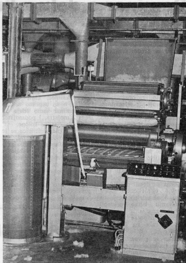
Mikalnik Platt z direktnim dovajanjem prediva.
