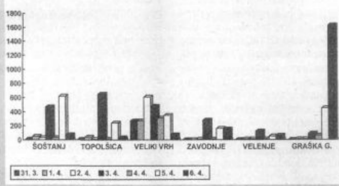
MAKSIMALNE POLURNE KONCENTRACIJE SO 2 od 31. marca do 6. aprila 1997
