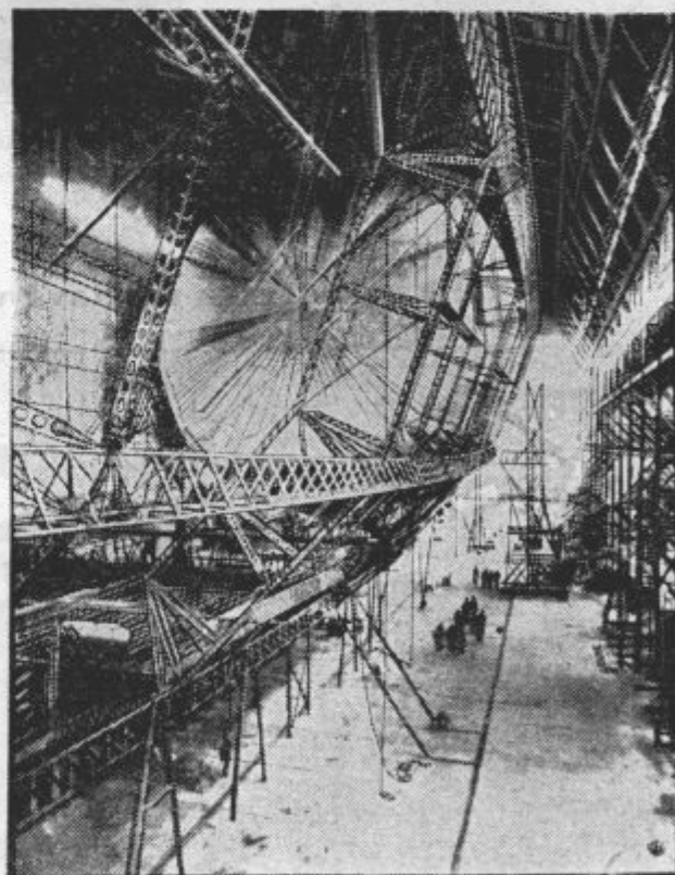
Obod zrakoplova »R 101« v gradnji
