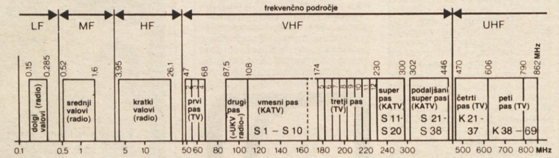
DEL VALOVNE LESTVICE – POJASNILA K FREKVENČNIM PODROČJEM:
