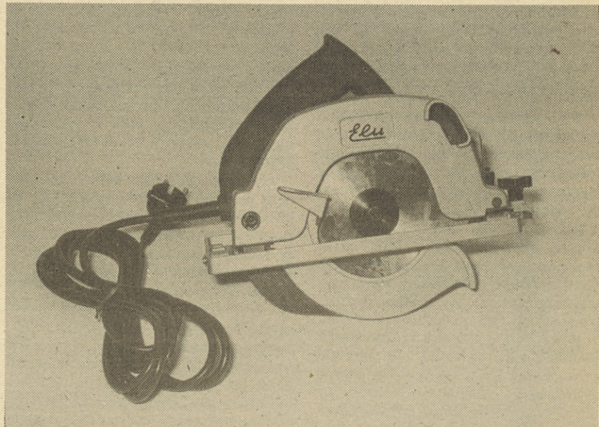
Nova krožna žaga, ki jo TOZD ERO izdeluje za nemško firmo ELU in jo bo mogoče kupiti tudi na domačem trgu.
