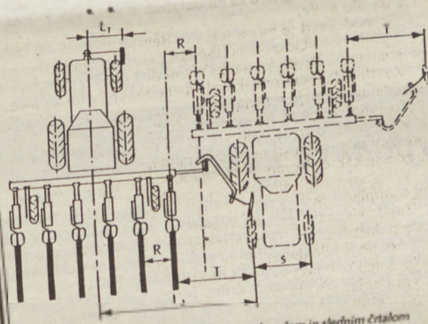
Sejalni agregat, opremljen s slednim kazalom in slednim črtilom
