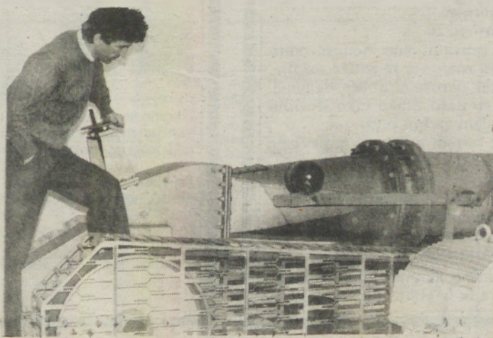
Generator v hidroelektrarni Majde Kurbus v Lovrencu na Pohorju se nenehno vrti in mesečno proizvede 35.000 kWh električne energije moči 380 voltov.
