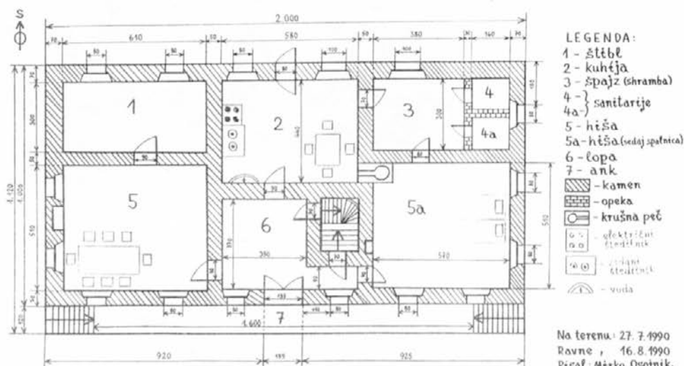
JASTROVNIK TLORIS PRITLIČJA HIŠE ZELEN BREG 13 M 1:100
