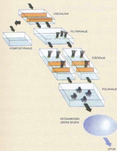
Schema delovanja rastlinske čistilne naprave (RČN)
