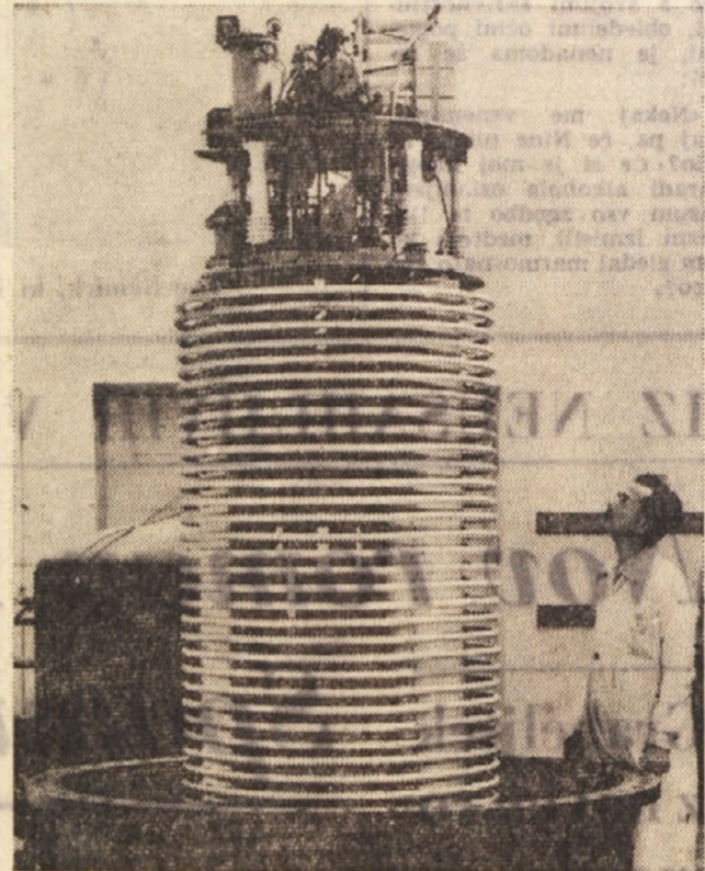
Notranjost akseleratorja Van der Graffa na ZMV. Sneta sta glava pospeševalnika in kotel, ki vzdržuje celo aparaturo pod pritiskom 10 atmosfer
