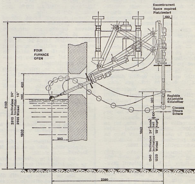
Shematski prikaz delovanja avtomatskega nabiralca stekla.
