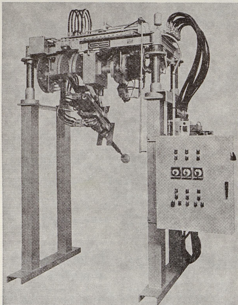
Avtomatski nabiralec stekla firme Guilhon Borhtelmy.
