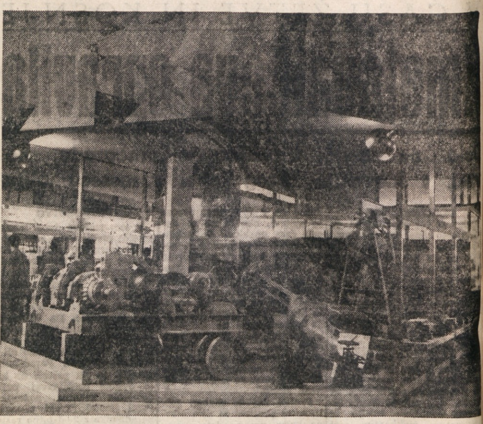
Pogled na jugoslovansko kolektivno razstavo v «Palači narodov». Na sliki vidimo razstavljene proizvode težke industrije, rezultat naporov nove tovarne «Litostroja» iz Ljubljane. Ob strani velik vodni zasun (v bistru vodovodna pipa) s premerom 70 centimetrov. V ozadju deli žerjavov, na levi pa maček z nosilnostjo 10 ton.
