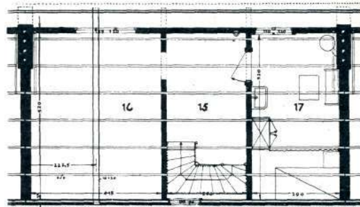
Iv. Vurnik: Načrt za uradniško enodružinsko hišo
