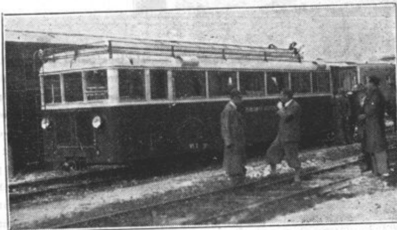
Motorni voz od strani; v njem je prostora za 40 potnikov
