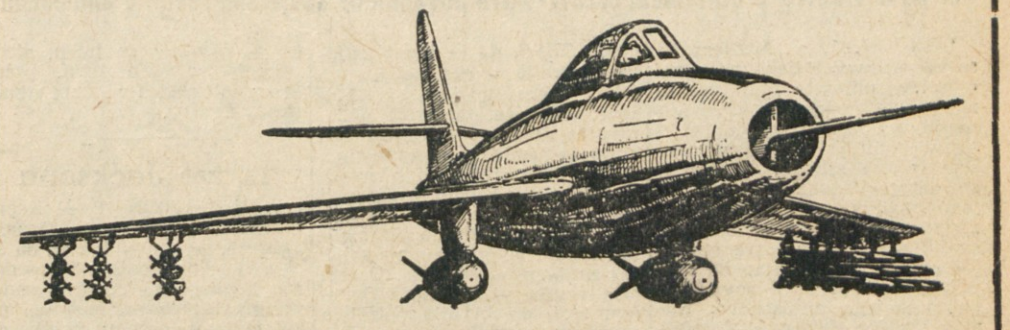
Republic F-84F je ena izmed poslednjih variant tipa F-84 «Thunderjet». Od prejšnjih modelov se razlikuje predvsem po puščastih krilih in repu. Varianta F-84F je izrazit predstavnik ameriških lovskih bombnikov. To letalo lahko nese poleg strelnega orožja še 18 raketnih projektilov 12,7 cm in 2 450kilski bombi.
