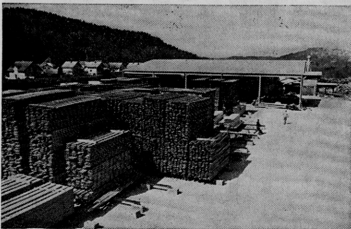
Del skladišča žaganega lesa s sortirno lopo v Podnartu
