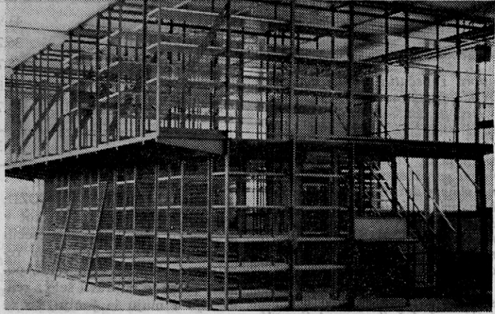
Regalno skladišče po montaži
