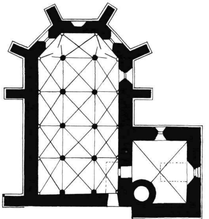
Sl. 4. Kapiteljska cerkev: kripta, talni načrt
