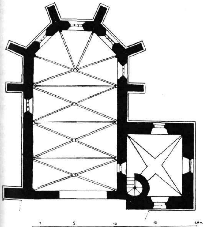
Sl. 2. Kapiteljska cerkev: prezbiterij, talni načrt
