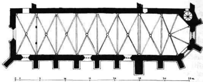
Sl. 3. Pleterske: samostanska cerkev, talni načrt
