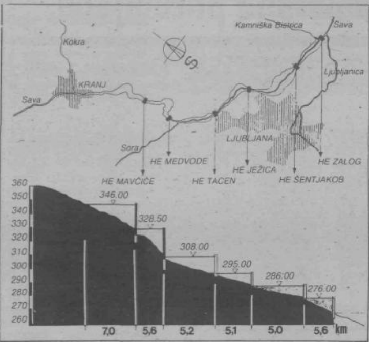
Skica prikazuje odsek Save med Kranjem in Zalogo pri Ljubljani. Tod naj bi bili člani bodoče verige pretočnih elektrarn. Na spodnjem delu skice so nadmorske višine, na katerih bo gladina Save za jezovi posameznih elektrarn.
