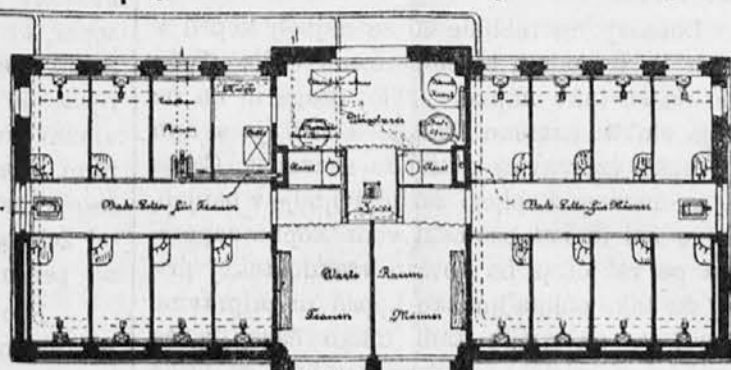
Grundriß
