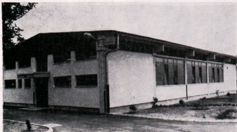
Vajenska šola v Zrečah, zgrajena po našem montažnem sistemu
