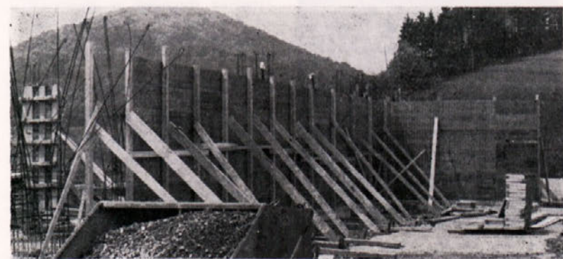
Opaz s ploščami LIP Bled po sistemu SAM porabo lesa zmanjšuje
