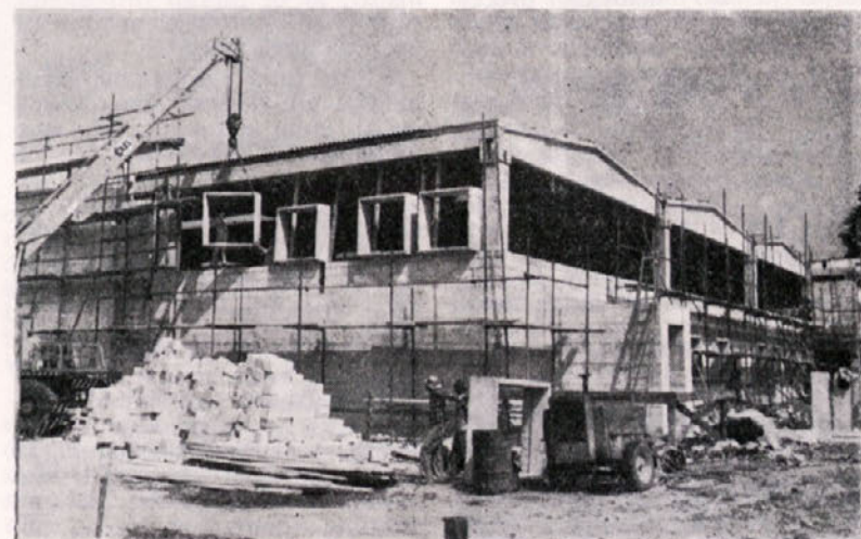
Montaža betonskega okenskega okvirja na hali »Lesnina« v Levcu
