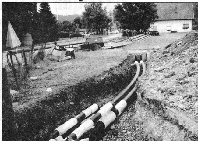
Priklop na obstoječo toplovodno instalacijo pri zdravstvenem domu (foto: Ciril M. Sem)
