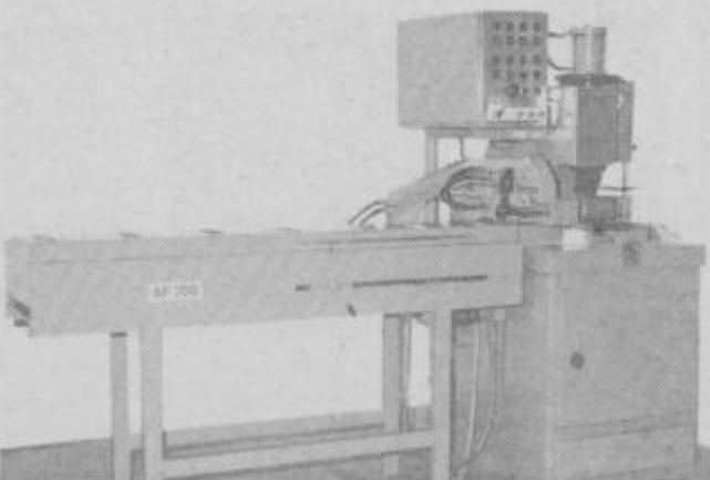
Avtomatska žaga za hladen razrez, ki so jo v Kovinarstvu Ljubno razvili za kovinsko-predelovalno industrijo.
