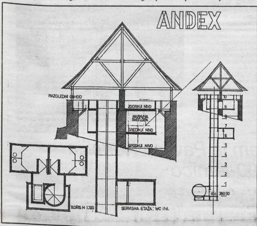
Prerez ureditve Stražnega stolpa, kot jo predlaga v svojem projektu prof. dr. Fedja Košir.
