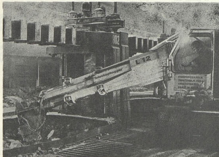
Izkop elektrolitske peči
